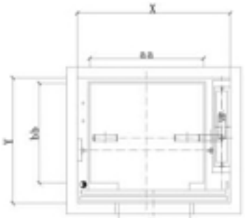
План шахты
