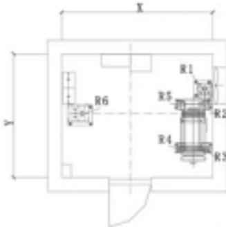
План машинного помещения
