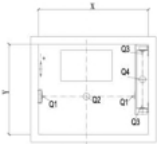
План приямка
