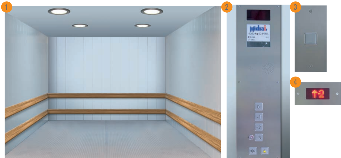
1. Кабина QHG. 2. Панель управления в кабине. 3. Панель управления на этаже. 4. Указатель направления движения лифта, расположенный на этаже.
