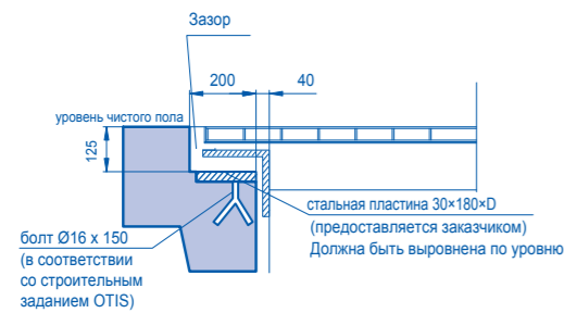
СТАНДАРТНАЯ ОПОРА
