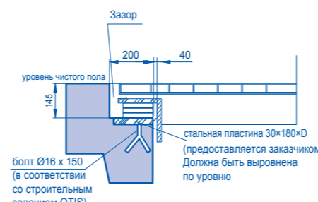
ОПОРА С АНТИВИБРАЦИОННЫМИ РЕЗИНОВЫМИ ПОДКЛАДКАМИ
