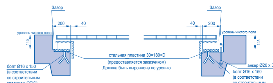
ОПОРА С ТЕФЛОНОВЫМИ ПОДКЛАДКАМИ ДЛЯ СКОЛЬЖЕНИЯ
