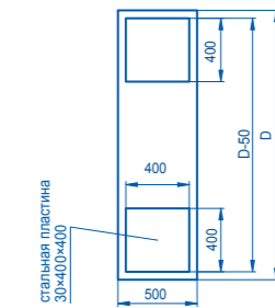
Промежуточная опора
