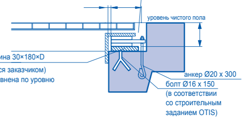
ОПОРА С ТЕФЛОНОВЫМИ ПОДКЛАДКАМИ ДЛЯ СКОЛЬЖЕНИЯ
