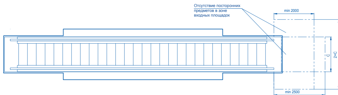
ВХОДНАЯ ПЛОЩАДКА С КОНТАКТНЫМ МАТОМ (для режима прерывистой работы)
