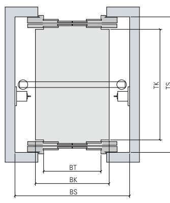
Два входа в кабину Центральное открытие (четырёхсекционная) C4
