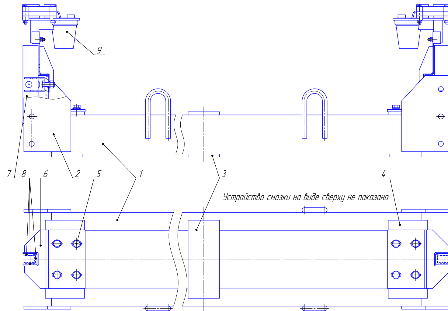
1 – швеллер; 2 – косынка; 3,4 – пластины; 5 – болт; 6 – кронштейн; 7 – корпус башмака; 8 – вкладыш; 9 – устройство смазки
