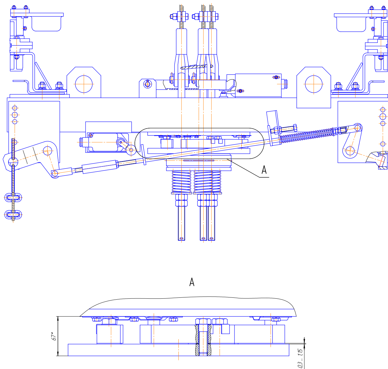
Рисунок 4.1.2 – Балка верхняя на трех тензодатчиках
