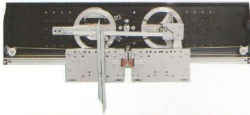
Tam Otomatik Merkezi 2 Panel Kabin Operatörü Full Automatic 2 Central Panels Cabin Operator полностью автоматический 2 панели центральных операторов кабины
