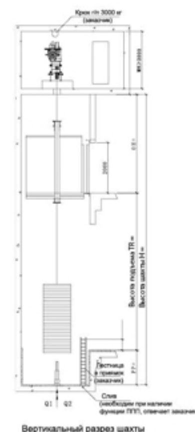
Вертикальный разрез шахты
