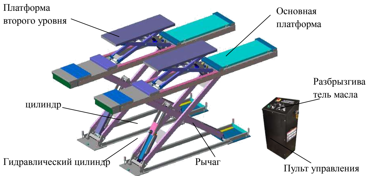
Рис. 1 Структура подъемника
