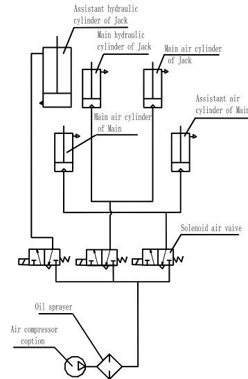
Рис.10-2 Принцип воздушной системы
